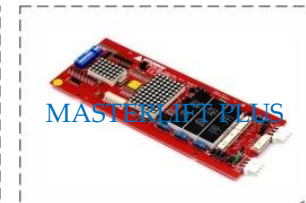
HIPD-CAN V3.2 Hyundai плата дисплея под заказ Арт: 0084
